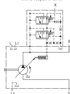
Схема гидравлическая
